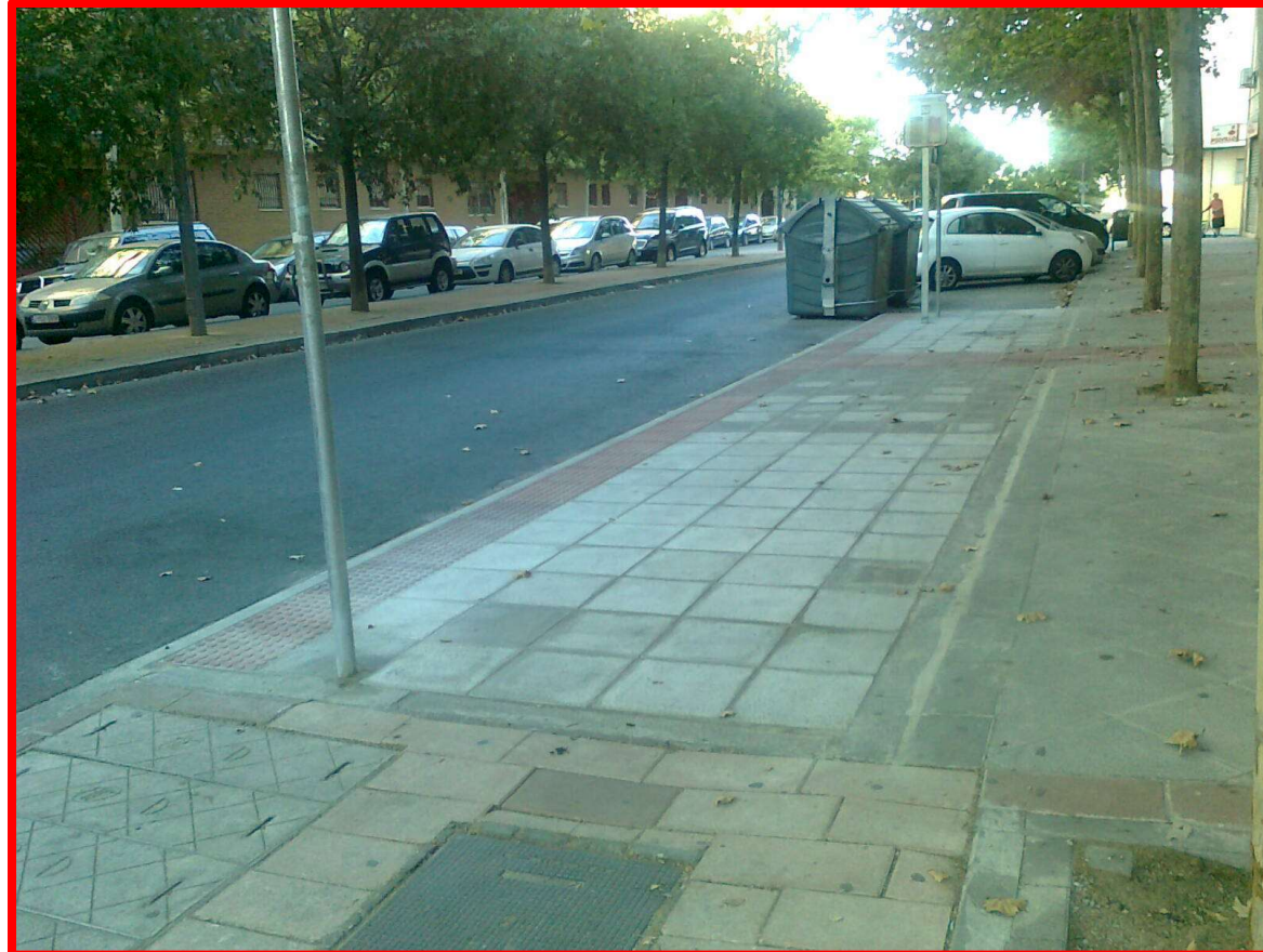
Construcción de plataforma parada Tussam C/ Baena (Julio)
